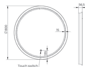
C-06-101MB Ø800 sa alu ramom 56,5mm LED matt black
