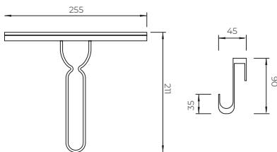
C-03-120 crni sa silikonskim držačem
