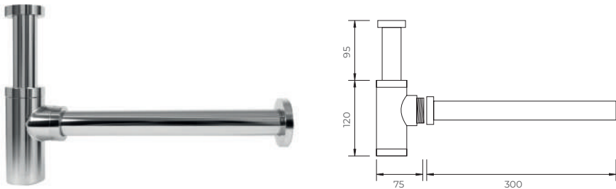
C-S-182 sifon za lavabo
