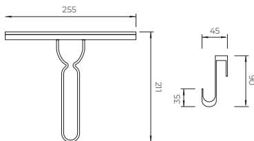
Linea C-03-109 hrom sa hrom držačem
