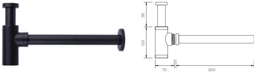
C-182B sifon za lavabo
