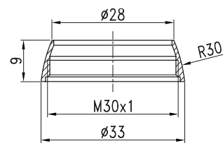
SP-COP30 Rozetna brušeno zlato
