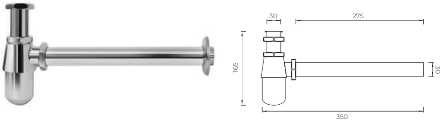
C-S-1004 sifon za lavabo
