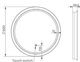
C-06-100MB Ø600 sa alu ramom 56,5mm LED matt black
