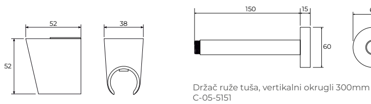
Držač tuš ručice C-05-5260
