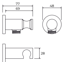
Konektor tuš creva sa držačem C-05-185
